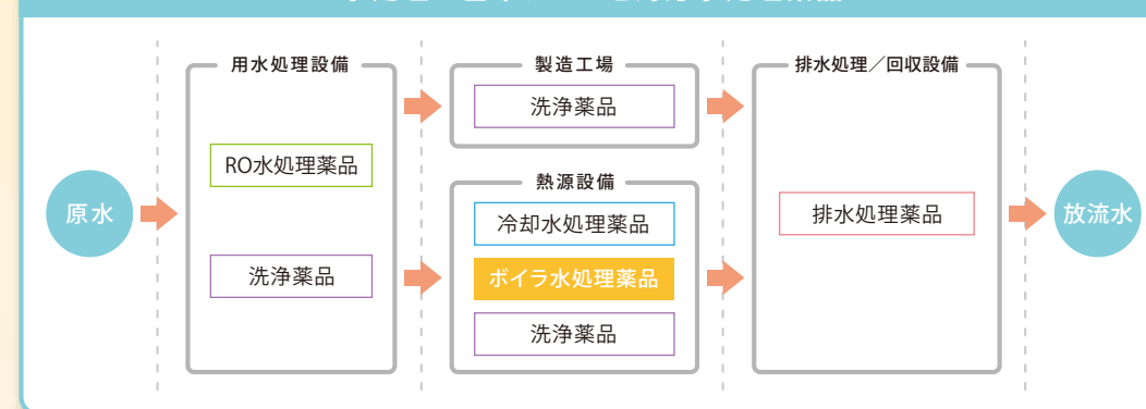
水処理の基本フローと対応水処理薬品
