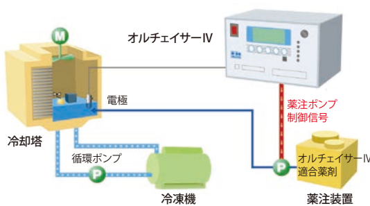
オルチェイサーⅣシステム構成図
